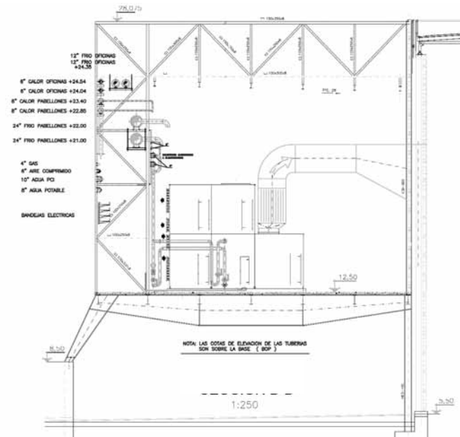
Detalle de las instalaciones de un pabellón (fuente: IDOM)
