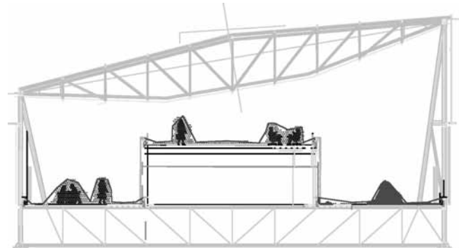
Esquema de tratamiento del aire de difusión por desplazamiento en el restaurante de pabellones
