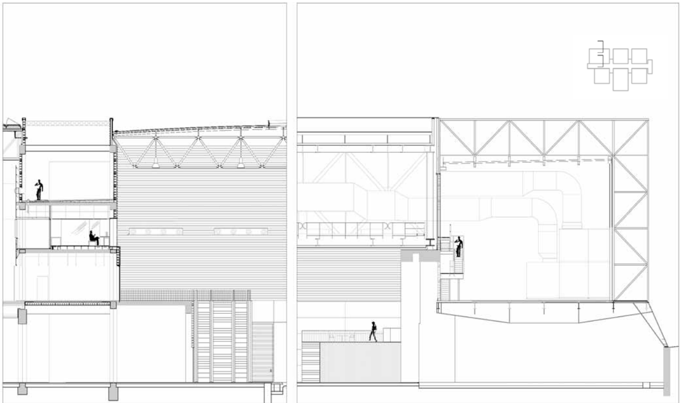
Sección con el espacio reservado para las UTAs de cada pabellón (fuente: IDOM)
