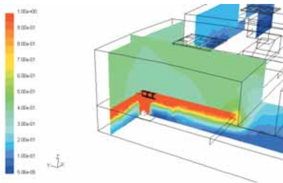
Análisis del funcionamiento del sistema de control de humos mediante técnicas de cálculo fluidodinámico (fuente: IDOM)
