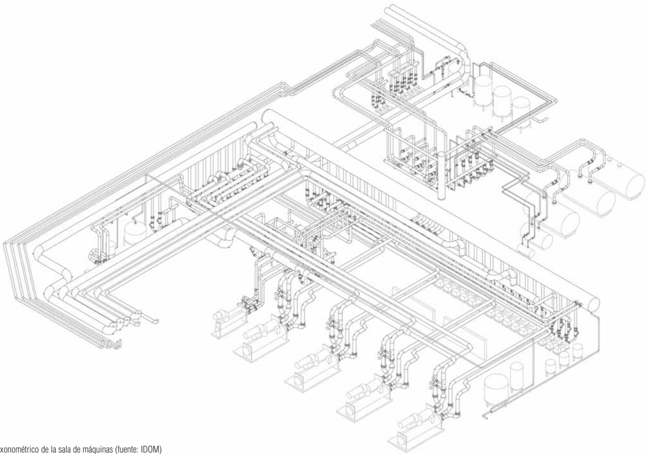
Axonométrico de la sala de máquinas (fuente: IDOM)
