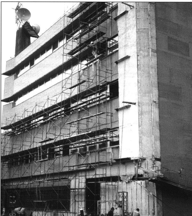
Ejecución de la fachada de chapa y colocación de los rastreles de madera en la parte baja para recibir el tablero estratificado. Comisaría para la ertzaintza de Bilbao
