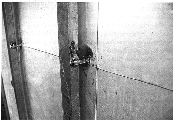
Detalle sujeción de rastreles para tablero estratificado. Aislamiento continuo.
