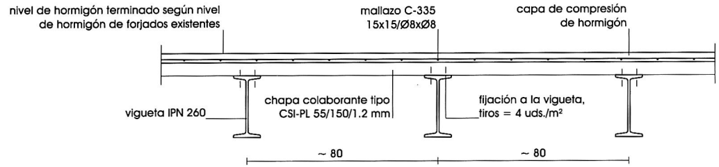
Sección 1
