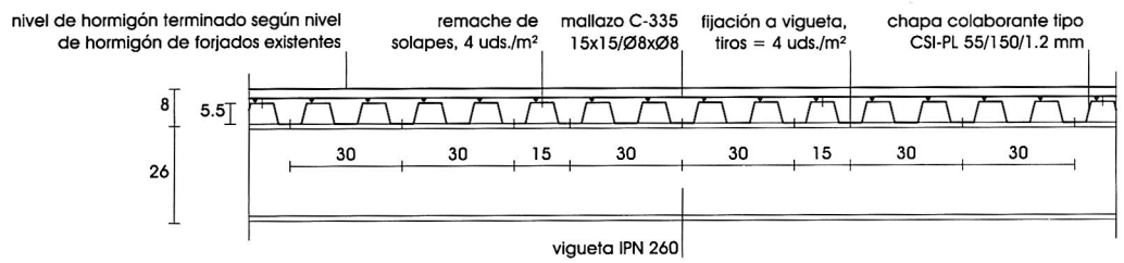
Sección 2
